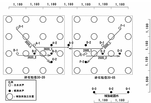
図1 砕石補強体および試験配置図
